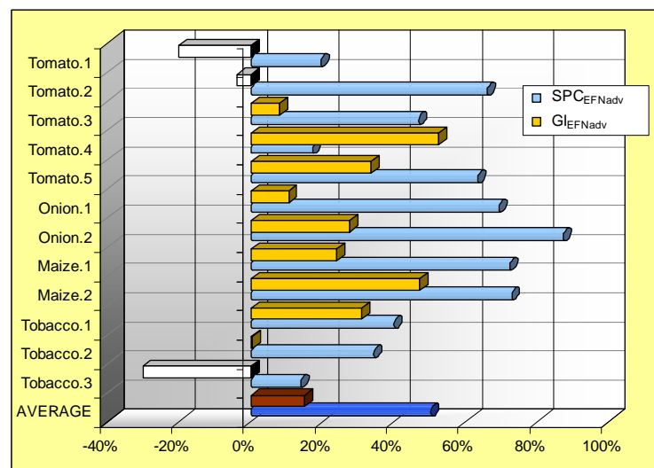
Fig. 9. Advantage of sprinkler on agronomic ( GI_{EFNadv} ) and economic ( SPC_{EFNadv} ) efficiency (Avantage de l'irrigation par aspersion sur le efficeine agronomique et économique)
