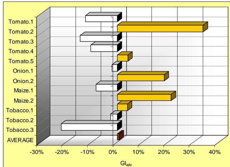
Fig. 2. Advantage of sprinkler on gross income (Avantages de l'irrigation par aspersion sur le revenu brut)
